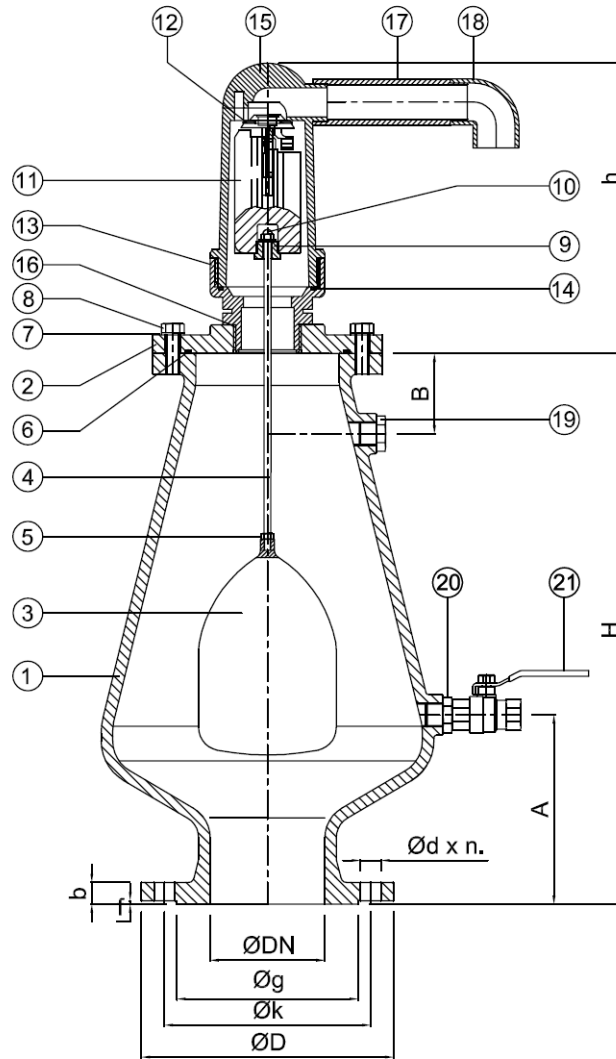
ISO 7005/2 BS EN 1092/2 PN16
